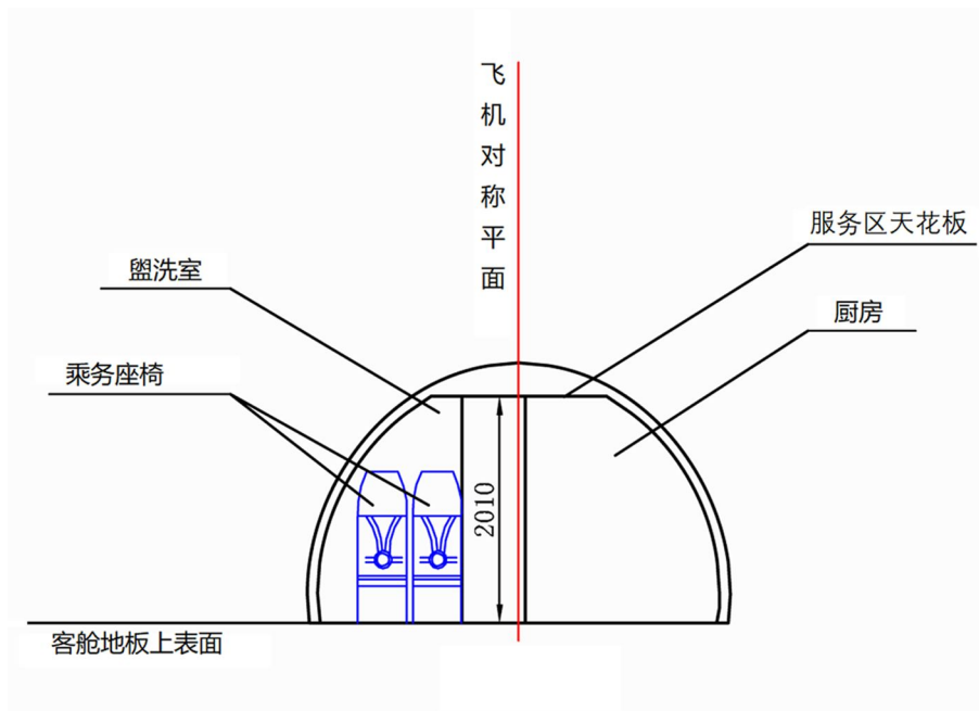
图 1 客舱截面图1(共1张 第1张)
