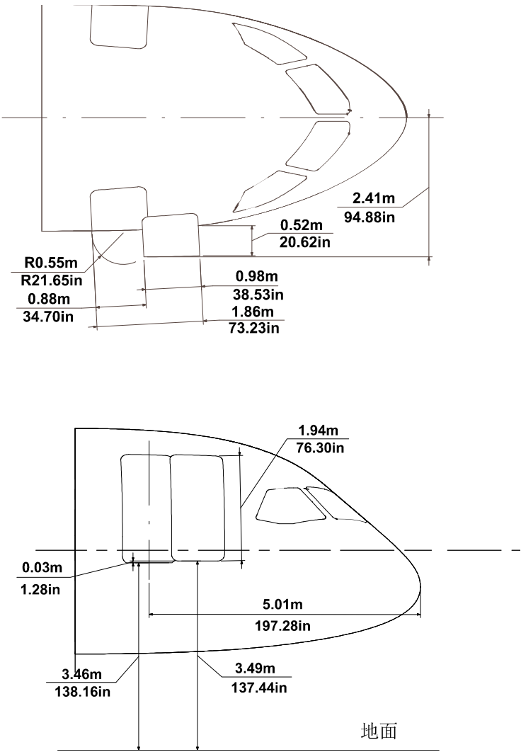
图 2 前服务门间距(共1张 第1张)
