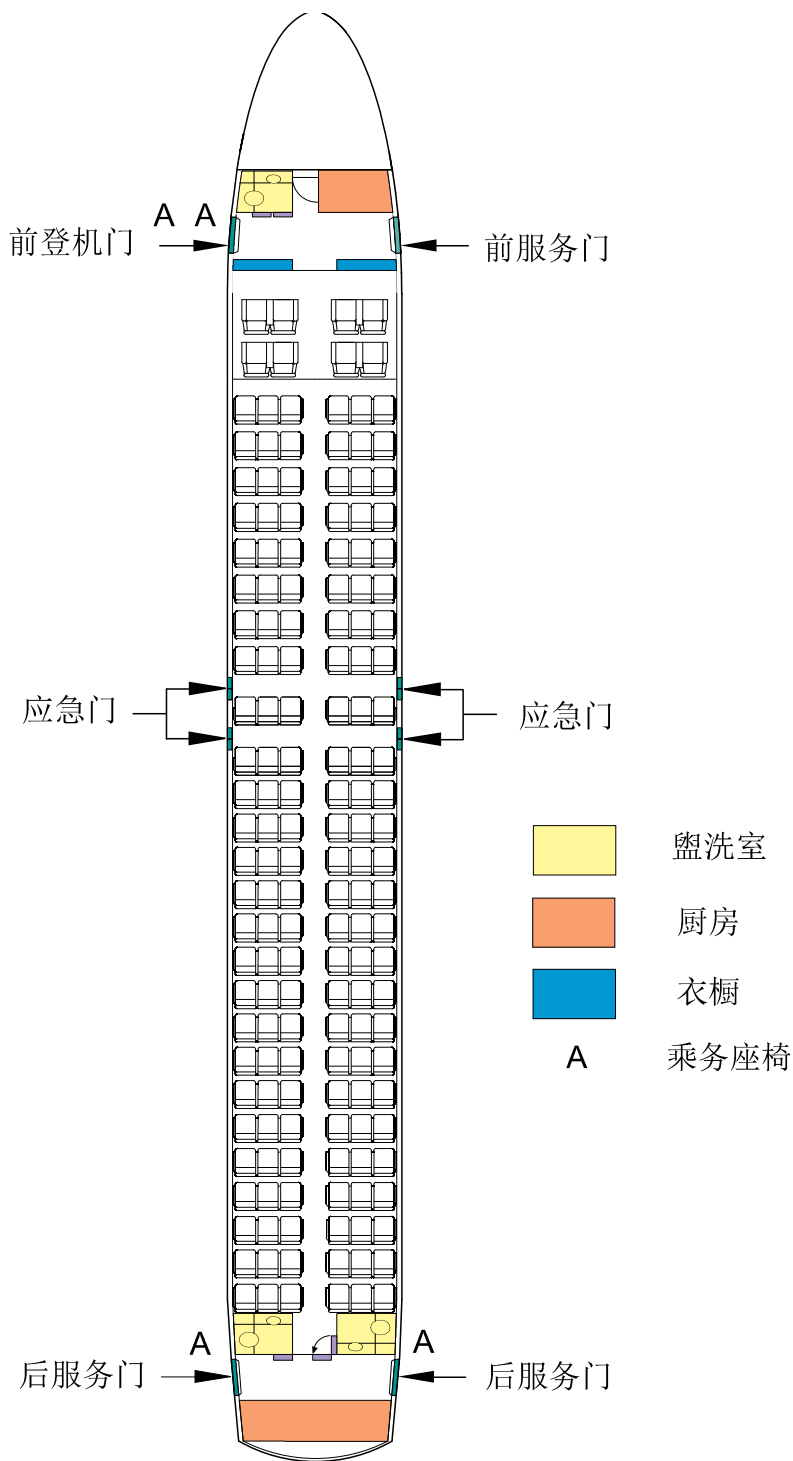
图 2 164座混合舱布局(共1张 第1张)
