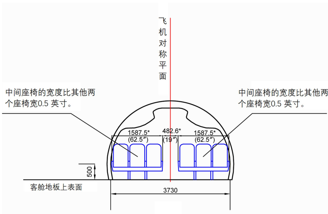
图 3 客舱截面图3(共1张 第1张)
