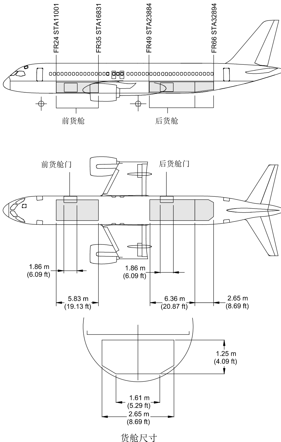
图 1 货舱数据 (共1张 第1张)
