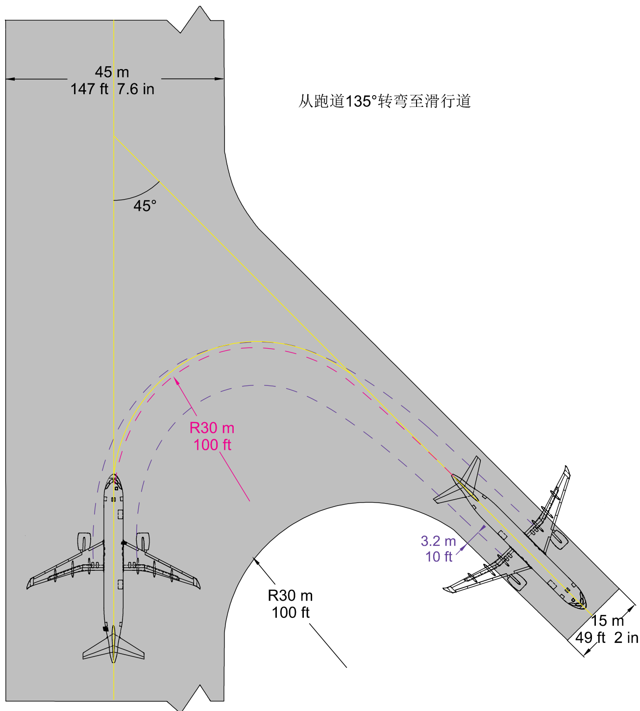
图 2 从跑道135° 转弯至滑行道(共1张 第1张)
