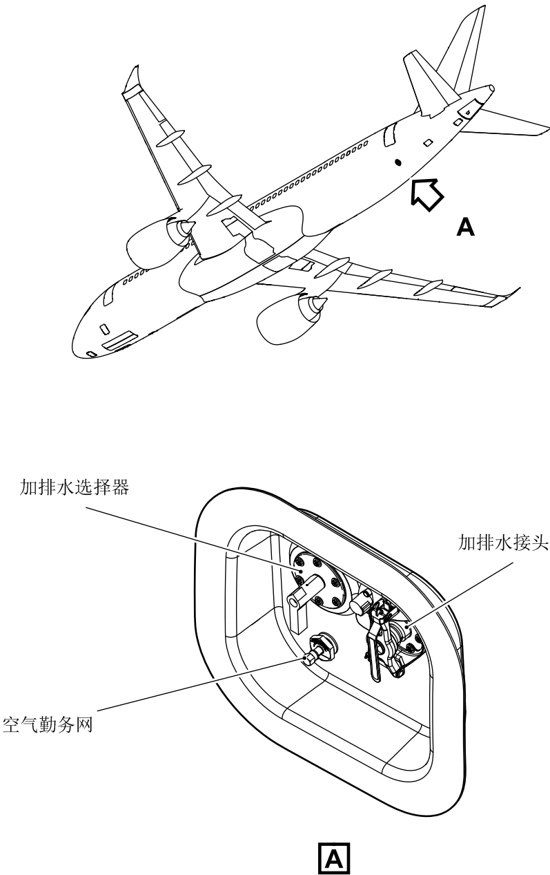
图 1 清水服务(共1张 第1张)
