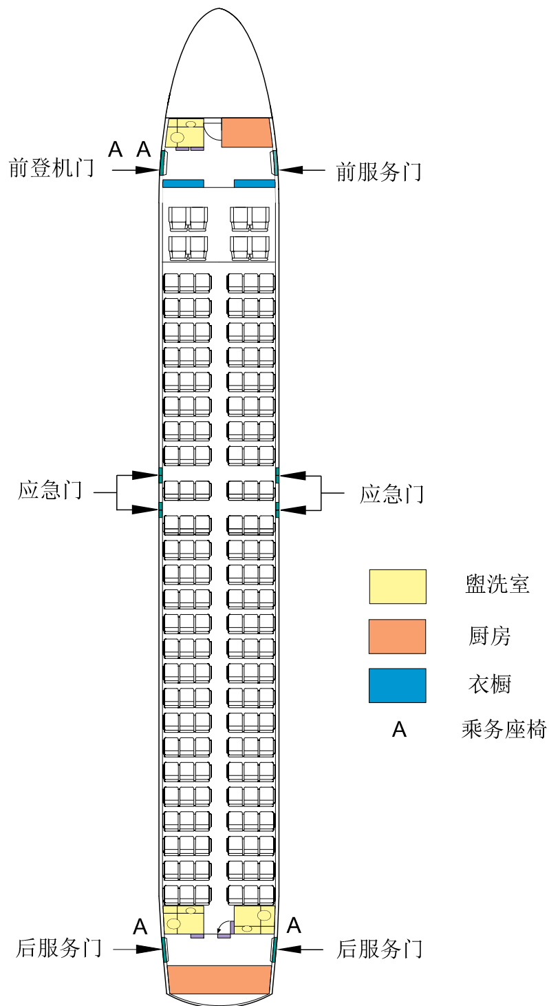
图 1 158座混合舱布局 (共1张 第1张)
