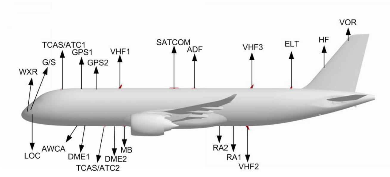
图 1 外部天线布置图 (共1张 第1张)
