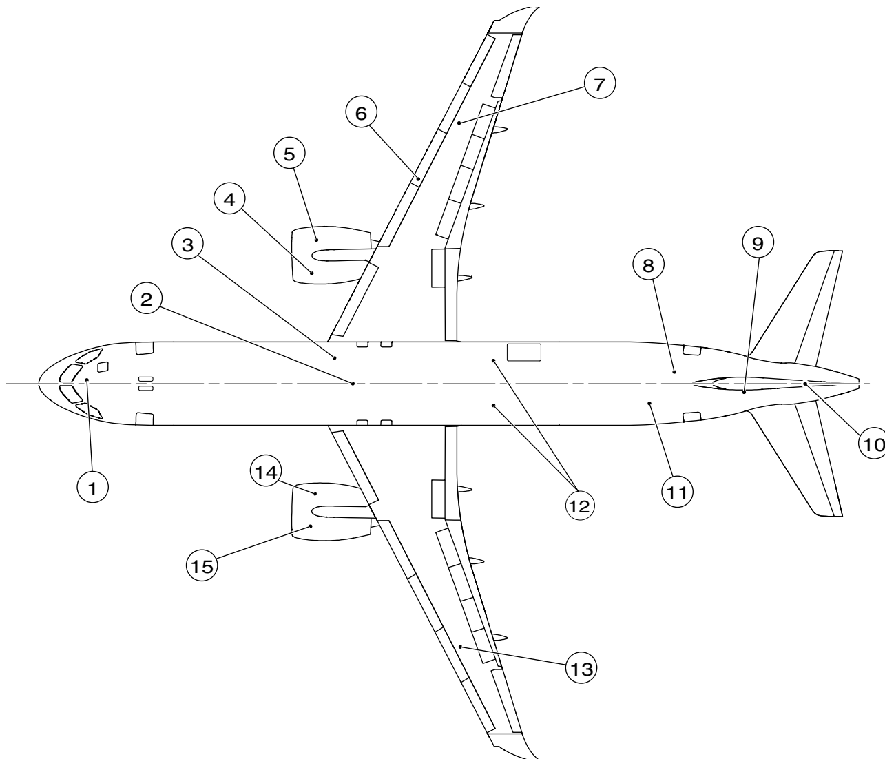
图 1 地面勤务接口 (共1张 第1张)
