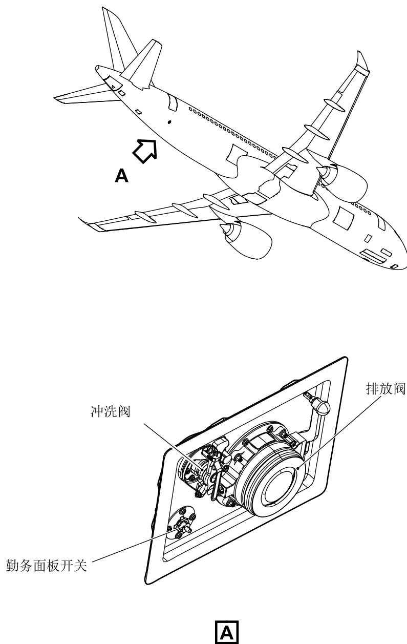
图 2 废水服务 (共1张 第1张)
