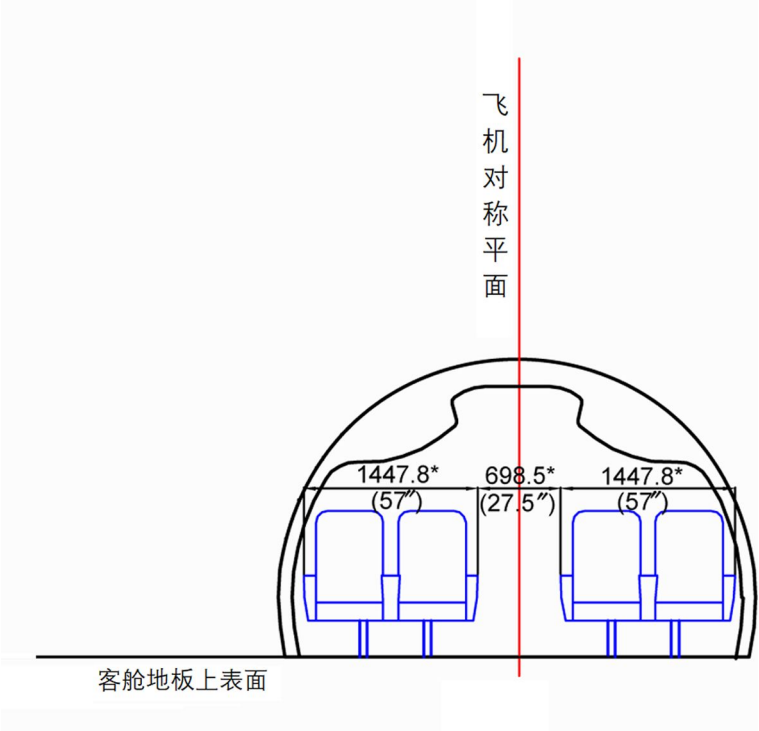
图 2 客舱截面图2(共1张 第1张)
